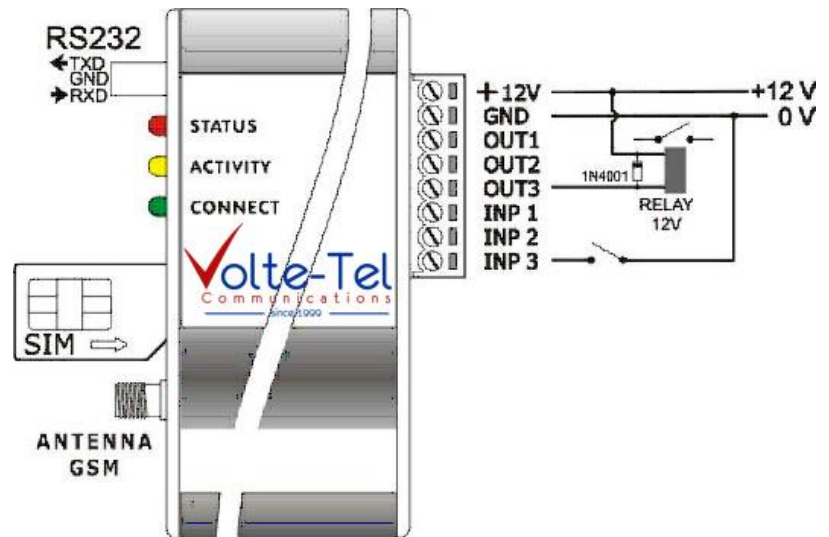
Σχήμα 1: Συνδέσεις του FCT-5 SMS
